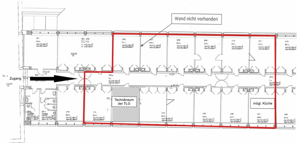
Grundrissauszug Bauteil B, 1. OG
